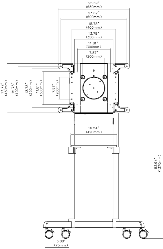
Vorderansicht
