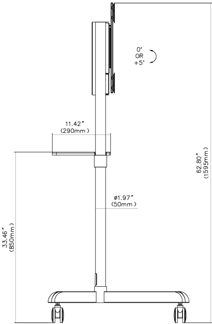
Seitenansicht
