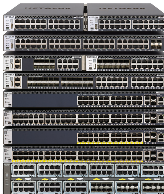
M4300-24X M4300-48X M4300-8X8F M4300-12X12F M4300-24X24F M4300-28G M4300-52G M4300-28G-PoE+ M4300-52G-PoE+ M4300-96X
