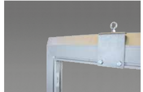
Montagepunkt für Abhängung.
