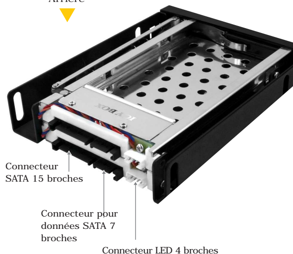
Arrière
